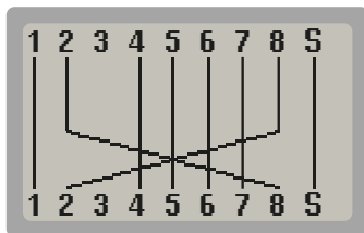
Vertauschung Pin 2 und 8, Unterbrechung Pin 3 Pin 2 and 8 twisted, break at pin 3
